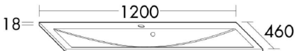
Dessin technique avec dimensions :
