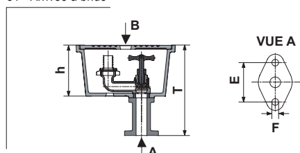
81 - Bouche d'arrosage non congelable arrivée à bride sans contre-bride
